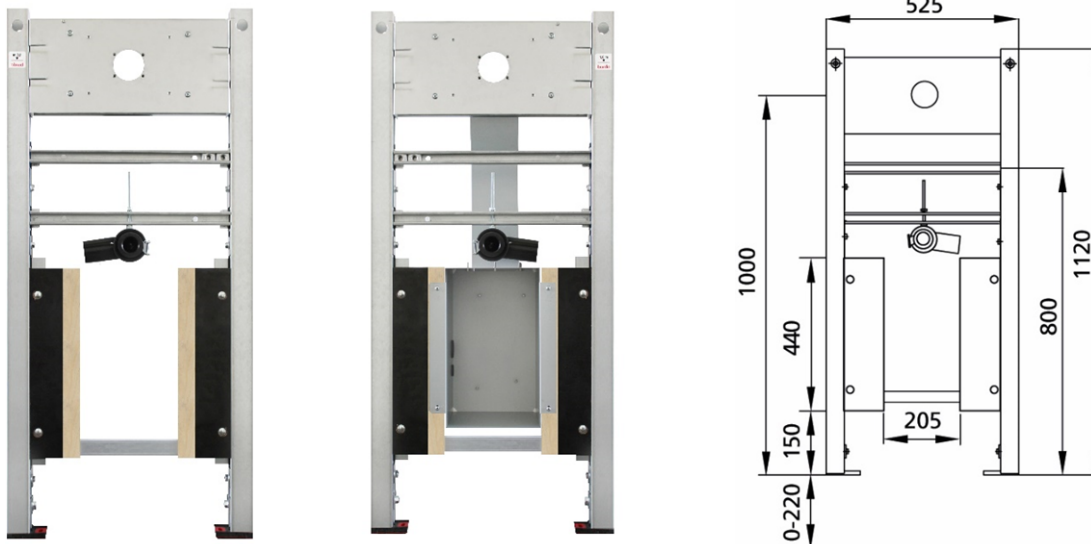
Darstellung mit bauseitigem Rohbaukasten
