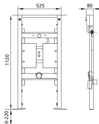
BS+ Urinal-Element mit Burda Universal Rohbauset Flowtronik item no. 214800
