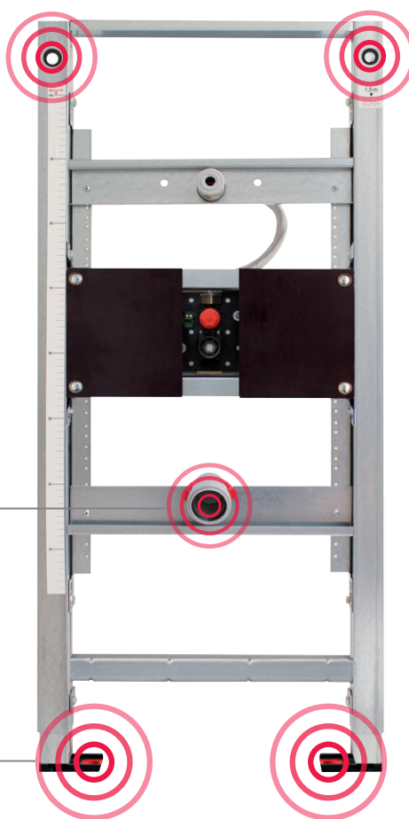
BS+ Urinal-Element mit Burda Universal Rohbauset Flowtronik item no. 214800
