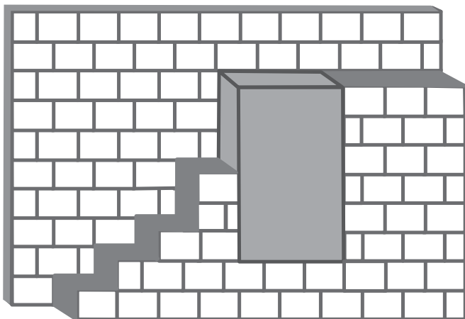
In Massivwand
