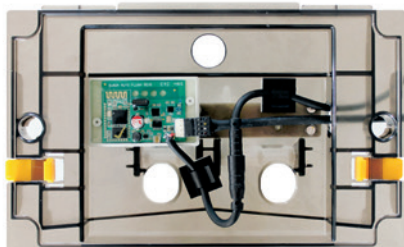
Spritzwasserschutzplatte inkl. Elektronik
