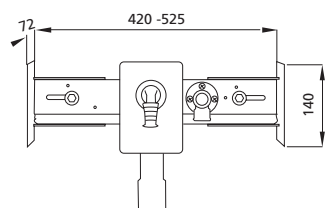
mit UP-Siphon WM und Wandscheibe 1/2". BS+ Traverse für Waschmaschine Art.-Nr. 216004 auf Wunsch auch mit Fremdpressanschlüssen
