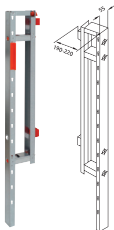
Typ 108 Bauhöhe 1080 mm Bautiefe 190-220 mm Art.-Nr. 667409
