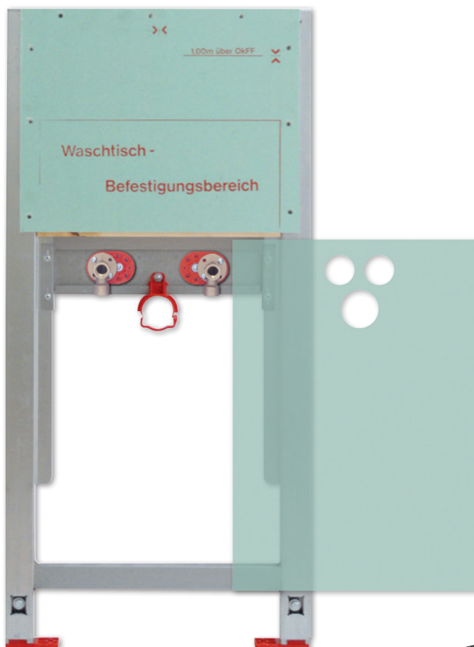
Santro WT-Modul für Standarmatur, BH 1080 mm Art.-Nr. 621258.00
