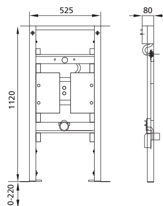
BS+ Urinal-Element mit Burda Universal Rohbauset Flowtronik Art.-Nr. 214800
