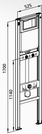
Traverse einstellbar von 770-1140
