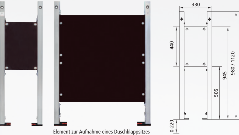
Element zur Aufnahme eines Duschklappsitzes
