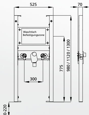
Beispiel UP-Siphon Haas OHA 3500
